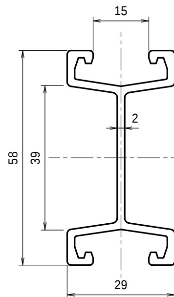
製品断面詳細図(1/1)
